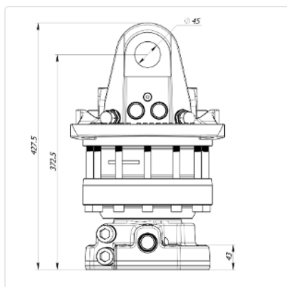
ГАБАРИТНЫЕ ЧЕРТЕЖИ РОТАТОРА FHR 16FD1
