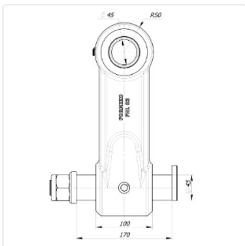
ПОДВЕСКА FHL 03 ГАБАРИТНЫЙ ЧЕРТЁЖ
